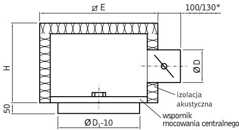
Standardowe wymiary skrzynek do nawiewników wirowych AWR-PO i AWK-PO
