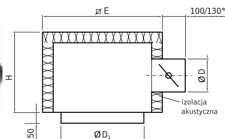
Standardowe wymiary skrzynek do anemostatów ANO
