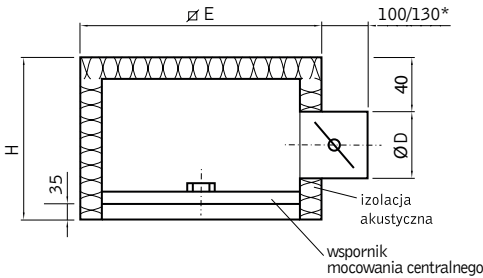
Standardowe wymiary skrzynek do nawiewników wirowych AWR-PK i AWK-PK
